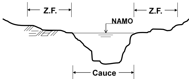
Figura 3. Esquema de delimitación de cauce y fajas de zona federal.
